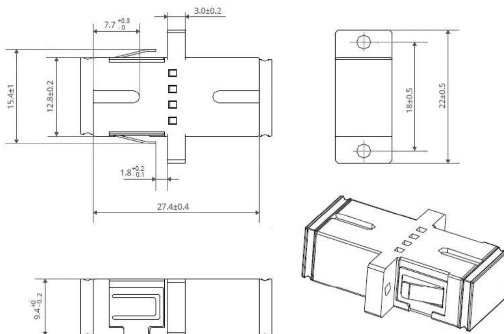
Desenhos técnicos:
